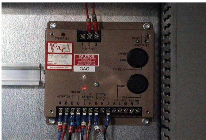
Régulateur de vitesse GAC type ESD 5550
